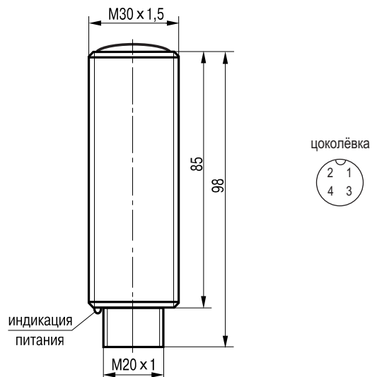
Габаритный чертеж
